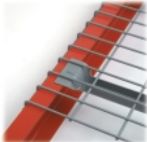
FLARE DECKING
